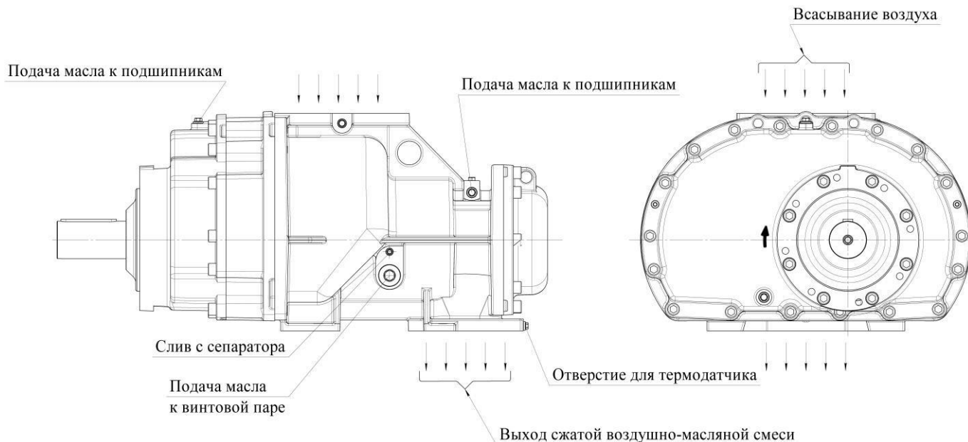
Рисунок 4 – Общий вид блока винтового VMX250G
